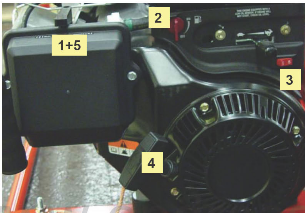
Рис. 4. : Пуск мотора
